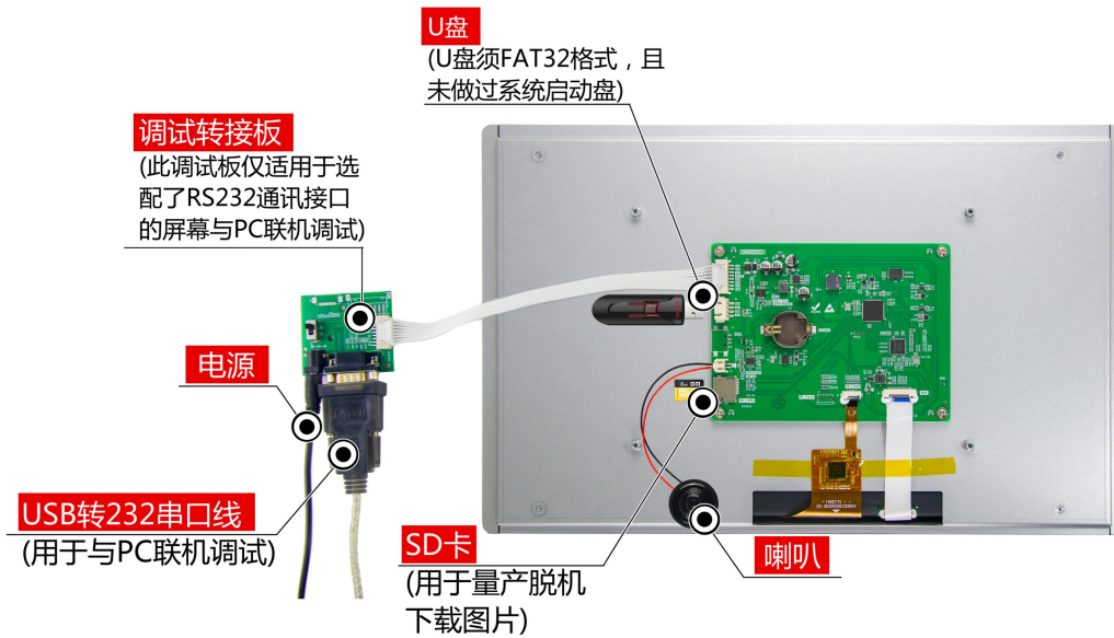
图 1-3 调试工具图
