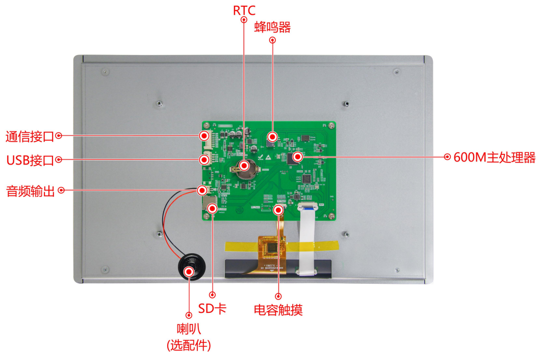
图 1-2 硬件配置图
