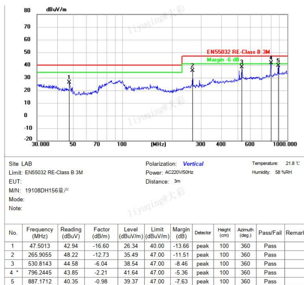
图 4-7 RE 测试垂直方向
