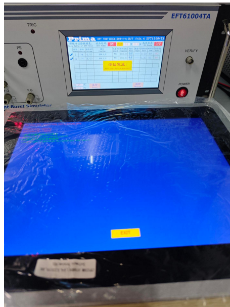
图 4-3 EFT 测试图
