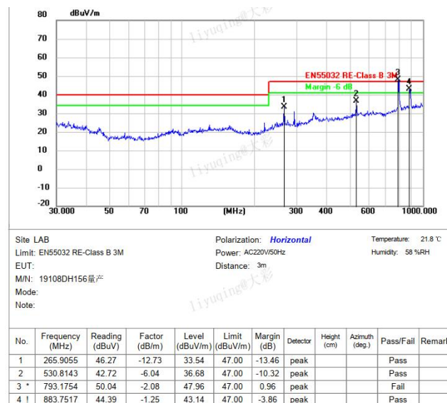
图 4-6 RE 测试水平方向
